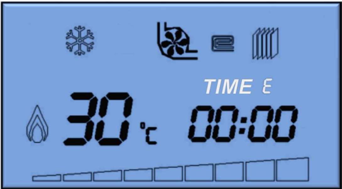
Рис 9. Индикация режима работы электрокотла по датчику уличной температуры.
