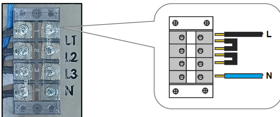
Рис. 11 Однофазное подключение
